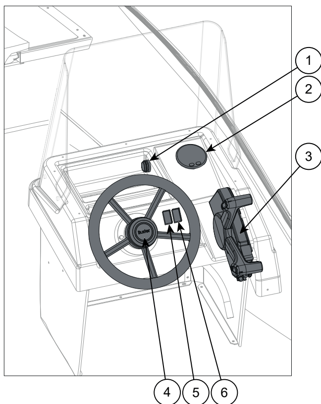
Figur 5.1 Förarplatsens kontroller på Buster XSr
