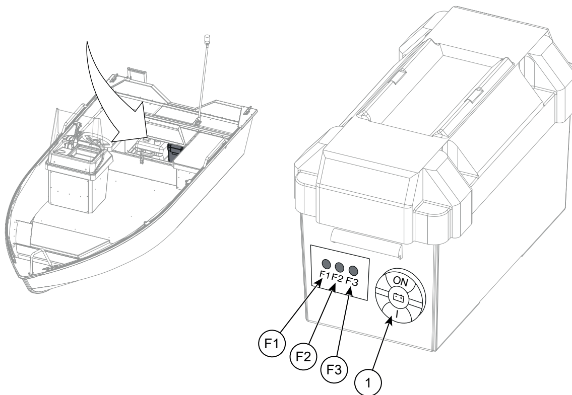
Figur 8.1 Buster XSr huvudströmbrytare och säkringspanel
