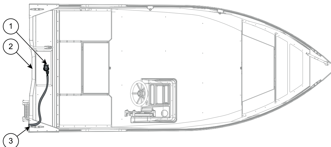
Figur 9.2 Buster XSr dräneringsutrustning
